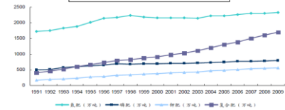
我国各种化肥历年施用量变化图
